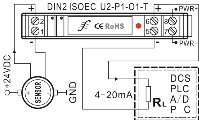
DIN2 导轨安装0-10V 转 4-20mA 接线图
