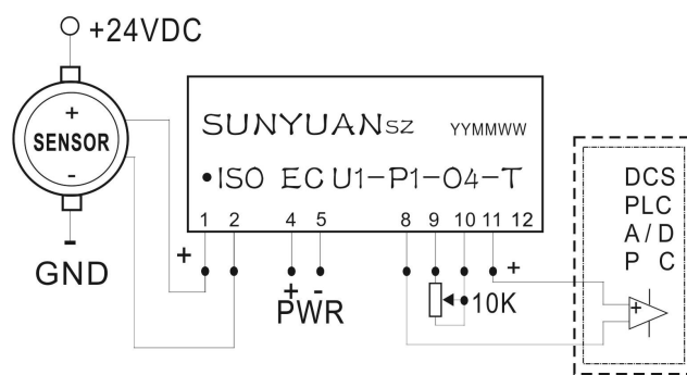
图4 电压输入/电压输出 (V/V) 隔离
