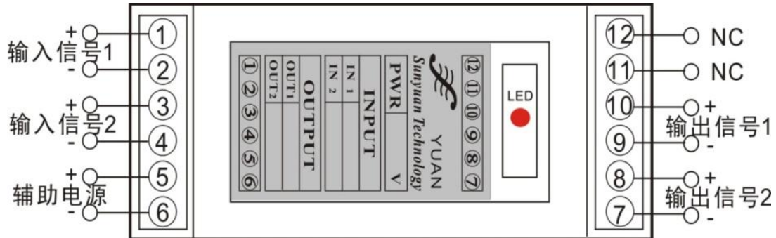
DIN 1X1 / 1X2 / 2X2 单/多路隔离放大器引脚功能及接线图
