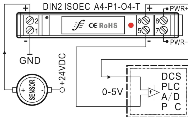
DIN2 导轨安装4-20mA 转 0-5V 接线图
