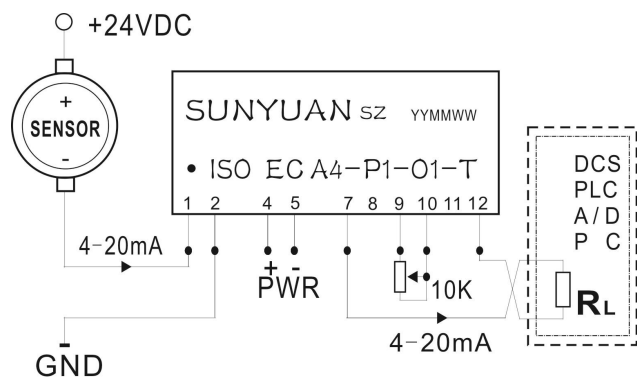
图1 电流输入/电流输出 (I/I) 隔离
