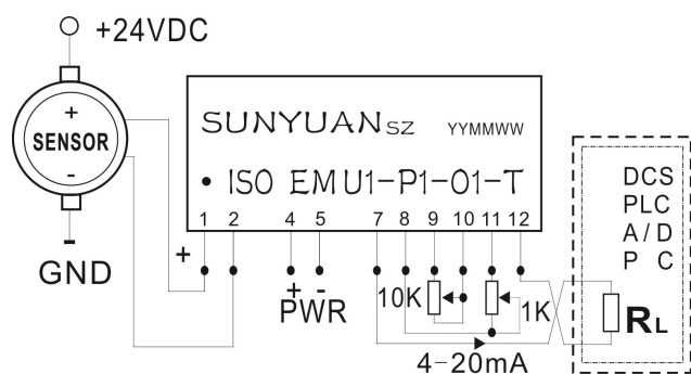
图3 电压输入/电流输出 (V/I) 转换
