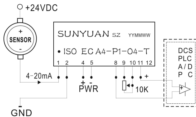
图2 电流输入/电压输出 (I/V转换)
