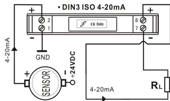
DIN3 ISO 4-20mA 小体积导轨安装隔离器接线图
